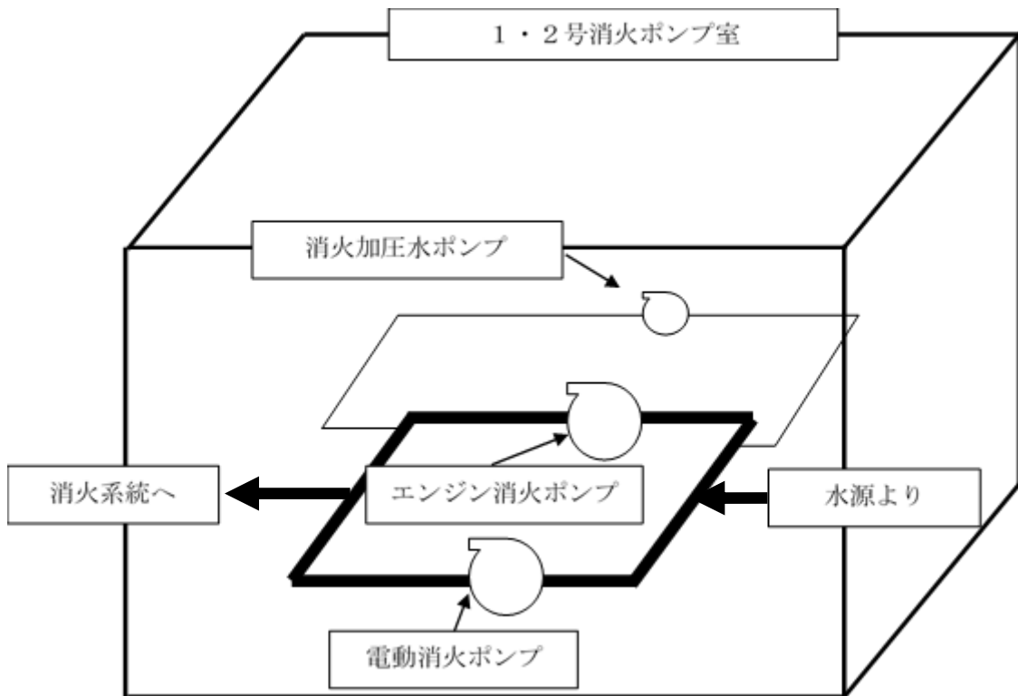
<ポンプ設置概要図>
