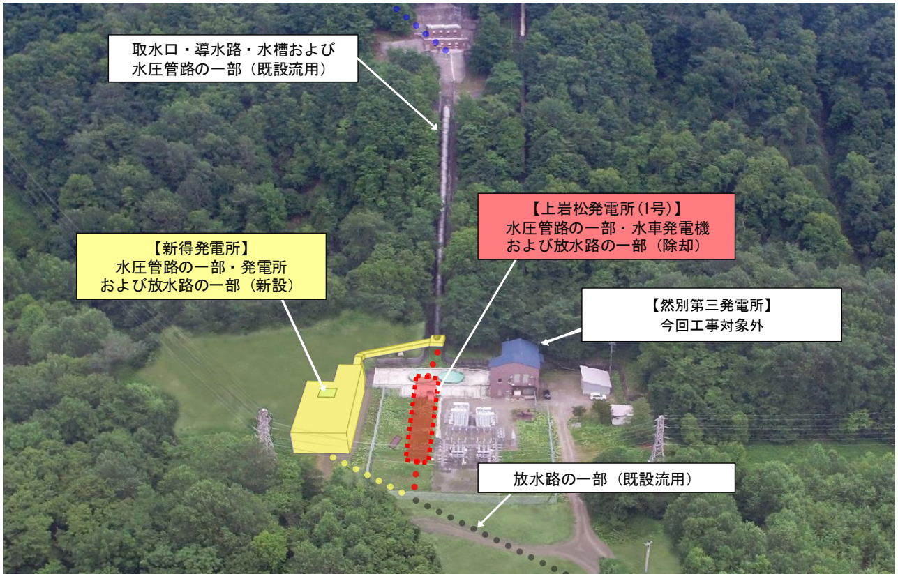
【 発電所外観 】
