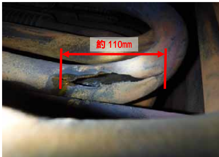
破孔管 (節炭器下部)
