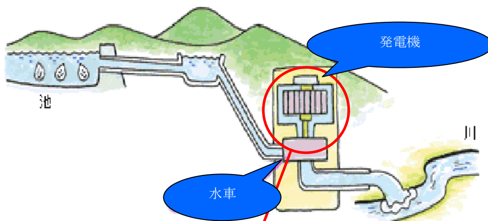
高見発電所 2号機 励磁装置系の概略図
