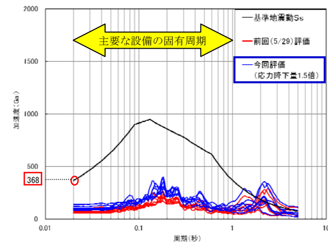
図-3 応答スペクトル図（鉛直方向）
