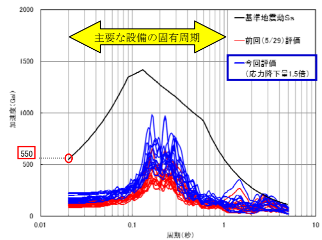
図-2 応答スペクトル図（水平方向）
