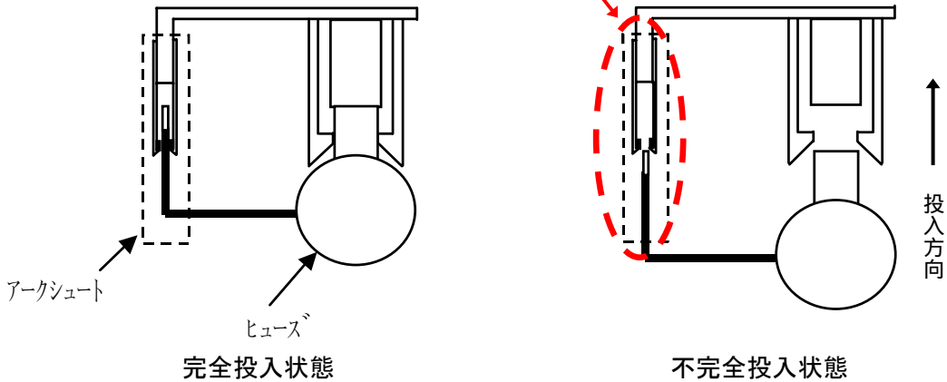
ヒューズ付スイッチ（上から見た図）
