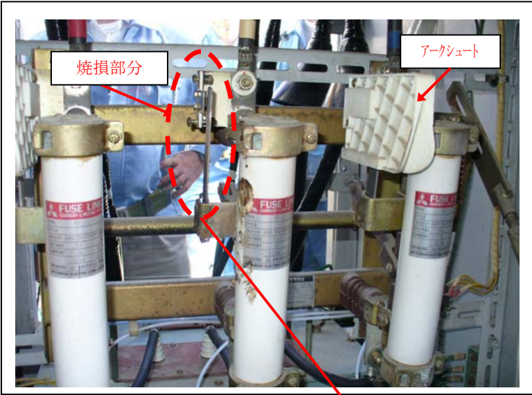
ヒューズ付スイッチ（上から見た図）
