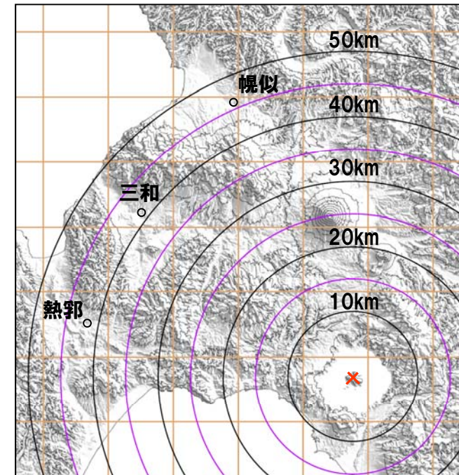
洞爺火砕流確認地点(当社地表地質踏査結果による)
