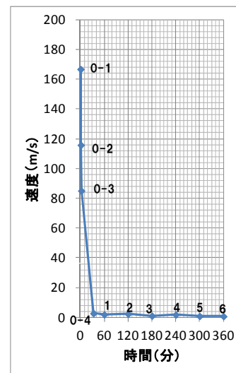
時間と火砕流速度の関係
