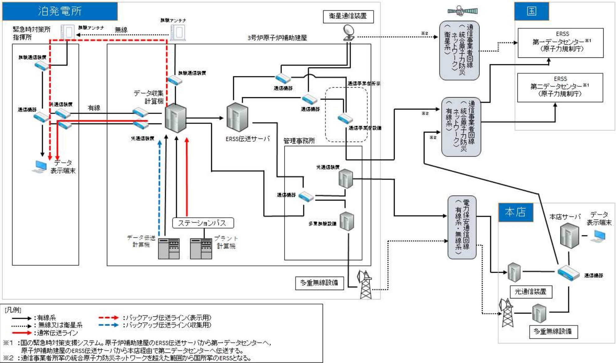
図5 緊急時対策所情報収集設備の概要
